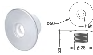
φ2" Face (Standard) Jet
