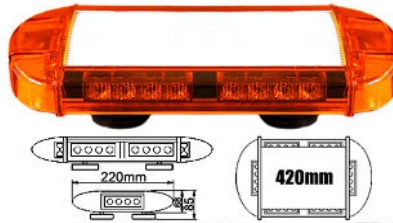
LED Warning Mini Lightbar LTL221
