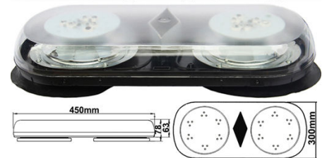
LED Warning Mini Lightbar LTL248
