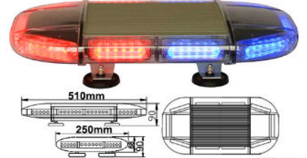
LED Warning Mini Lightbar LTL289
