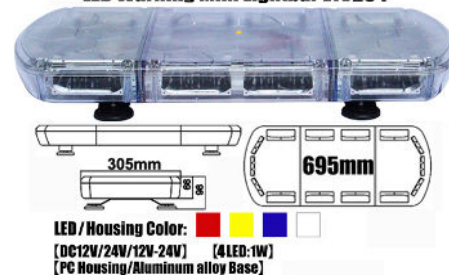
LED Warning Mini Lightbar LTL234
