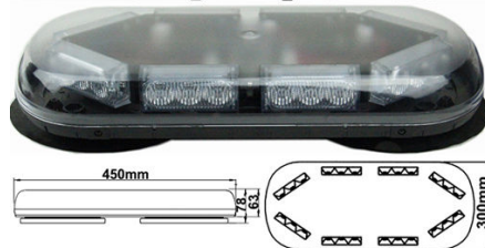
LED Warning Mini Lightbar LTL247
