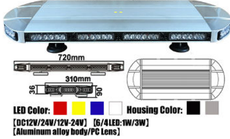
LED Warning Mini Lightbar LTL263
