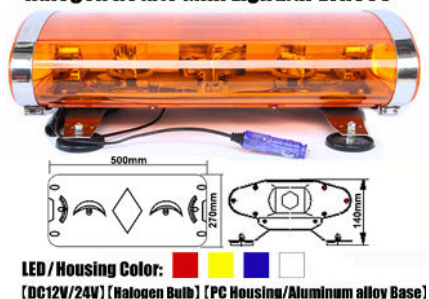
Halogen Rotate Mini Lightbar LTR506
