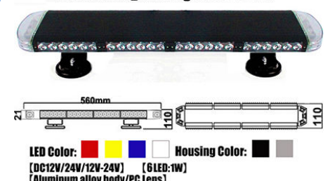
LED Warning Mini Lightbar LTL216
