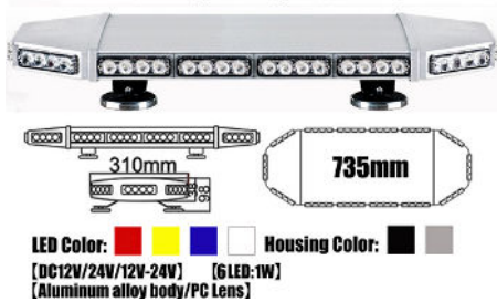
LED Warning Mini Lightbar LTL232B
