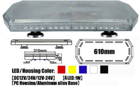
LED Warning Mini Lightbar LTL222
