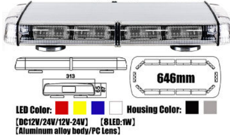
LED Warning Mini Lightbar LTL229A
