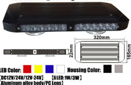
LED Warning Mini Lightbar LTL287
