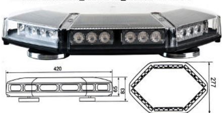
LED Warning Mini Lightbar LTL238
