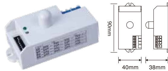
PS-RS12
