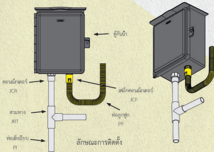
ท่อลูกฟูก PF และข้อแข็ง PI
