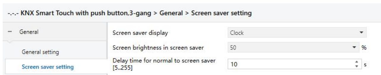
Fig.5.1.2 “Screen saver setting” parameter window
