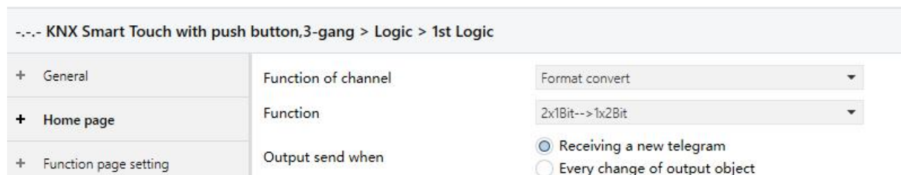
Fig.5.8.4 "Format convert" parameter window
