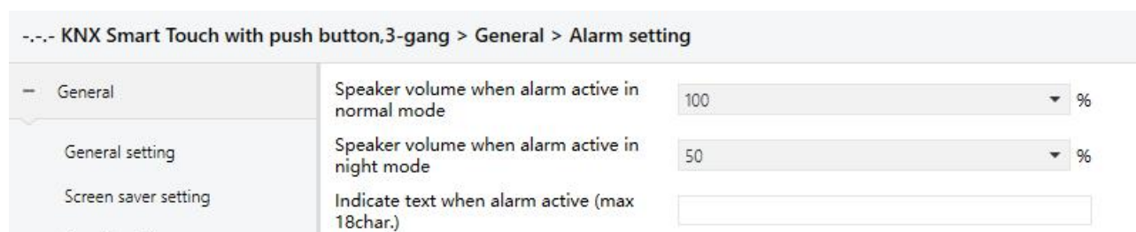
Fig.5.1.7 “Alarm setting” parameter window
