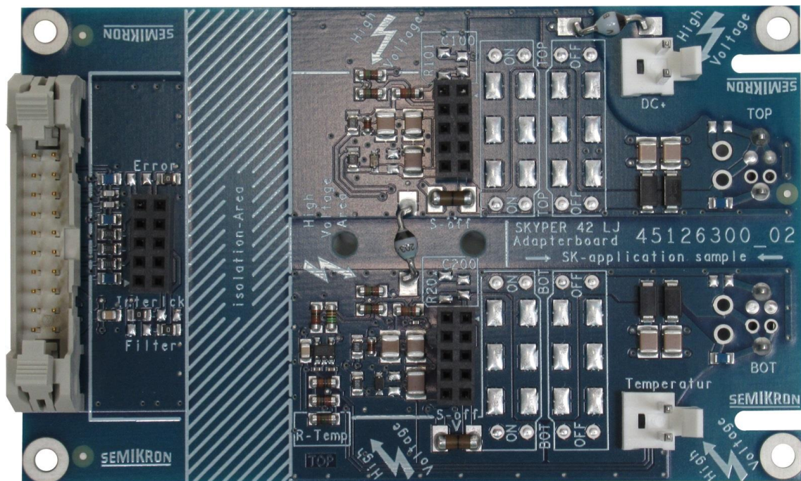
Figure 4: Board SiC Module SKYPER 42 LJ
